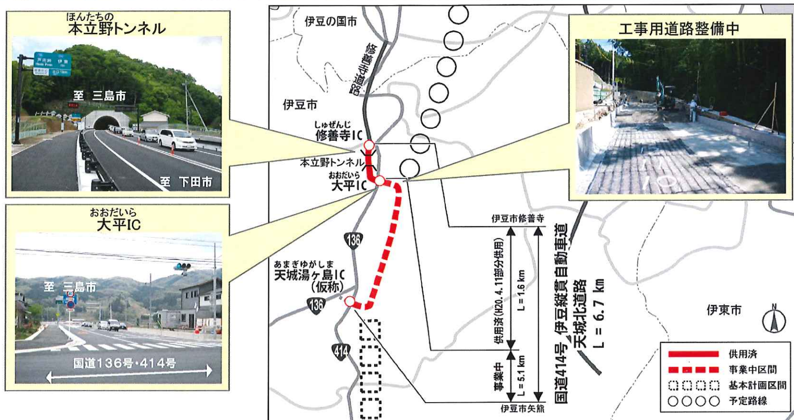
図8 天城北道路供用区間
